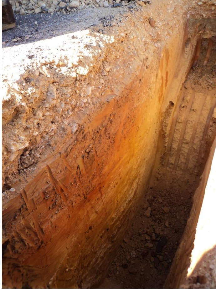
Photo 1 : Test Pit
